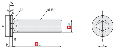
PSBN 六角孔型
