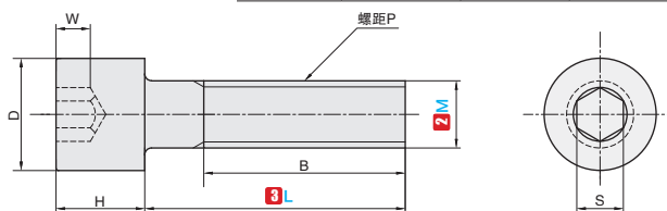
PSHQ 短圆柱头型
