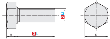
PBA 全螺纹型
