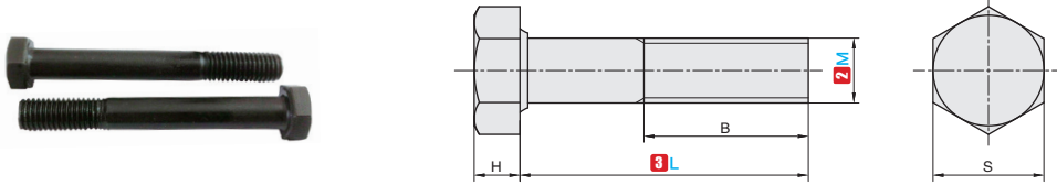
PBH 半螺纹型
