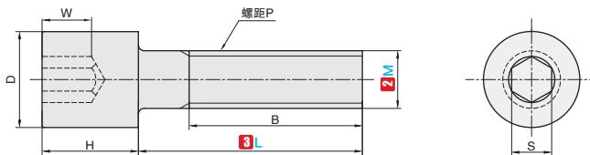
PSHC 圆柱头型
