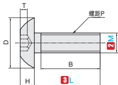
PSHF 平圆头型
