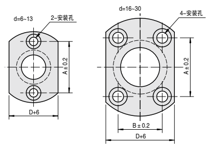
OFBTNZ 两边切割法兰型
