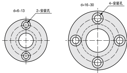
OFBTZ 圆法兰型
