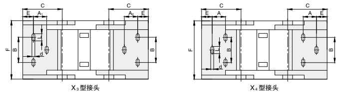
X 3 型接头
