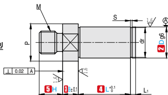
HCESND 螺纹长度选择型
