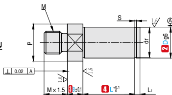
HCESNX 螺纹长度固定型
