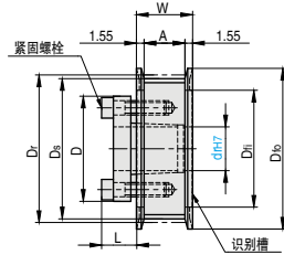
SET5F 标准型
