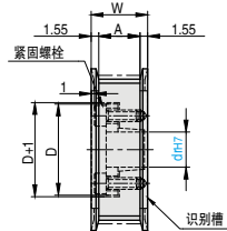
SET5G 沉孔型
