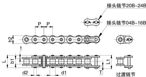
标准B系列链条
