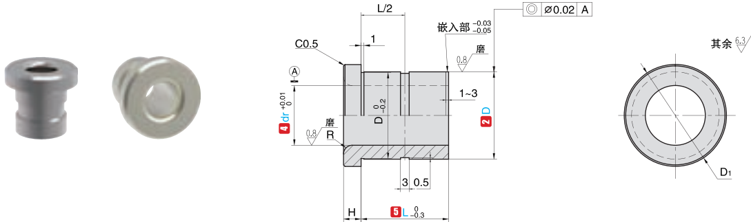
BGET 尺寸指定型
