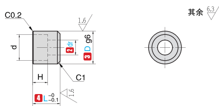
LDC 沉孔型
