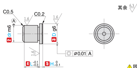
LDS 台阶型
