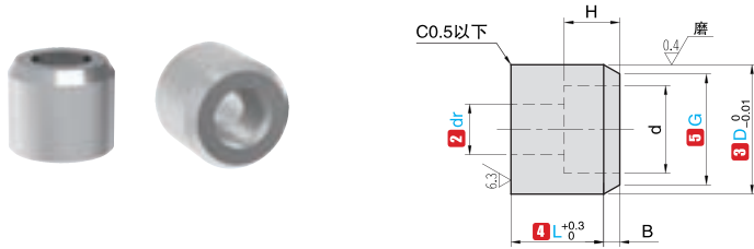
LLM 螺栓固定型
