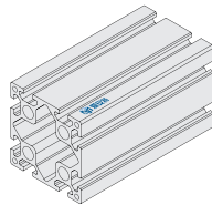
80x80-8 槽 重型
