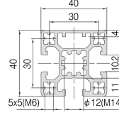
40x40-4 槽
