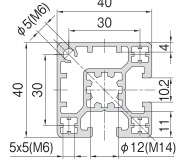
40x40-4 槽 轻型
