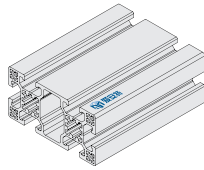
40x80-6 槽 轻型
