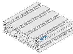
40x160-10 槽 重型
